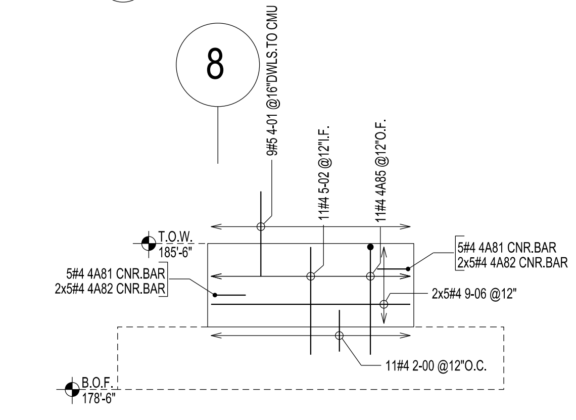
E3 CONCRETE WALL ELEVATION R104
